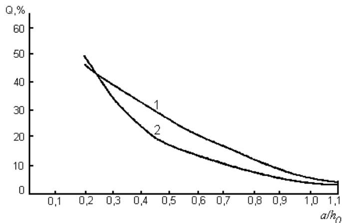
Рис.ПЗ.3. Зависимость доли перелившейся через обвалование жидкости
